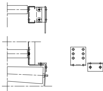
FR 100 – Skarv mellan rak bana och en kurva med längre rullar
