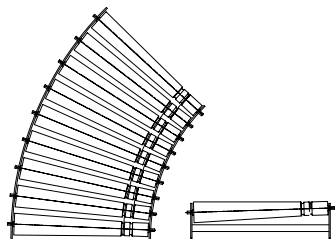
AX100 – Kurva, driven 45° med driverolls
