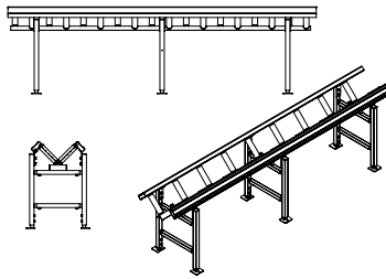
AX100 – Rullbana, odreven med rullar i 90°
