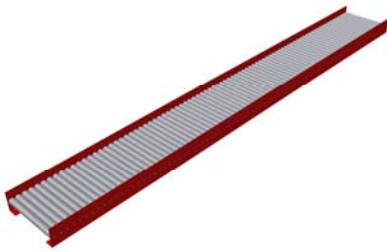
S50 – Rullbana, odreven. Rulldiam. 32 mm. Rulldelning 34 mm
