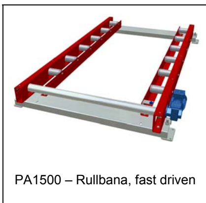
PA1500 – Rullbana, fast driven. Rulle till rulle drift. Rullar 5 mm över spant. Rulldiam. 89 mm
