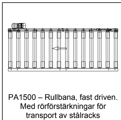
PA1500 – Rullbana, fast driven. Rulldelning 93,7 mm
