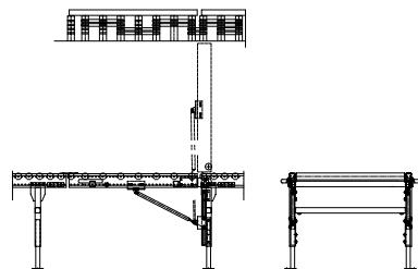
AX100 – Grind, rulle till rulle drift
