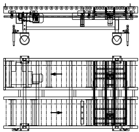
AX100 – Flyttbar robotmodul med fixering
