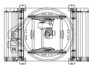
PA1500 – Vridmodul med kort kedjetransportör för vridning av 1/2-pall
