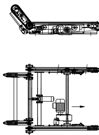
PA1500 – Kedjetransportör med tillbar ände för placering på vridmodul
