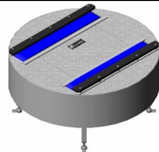
PA1500 Rostfritt – Vridmodul med 2-strängad plastlamelltransportör
