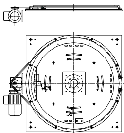
PA1500 – Vridmodul utan ben och med lös motorhylla
