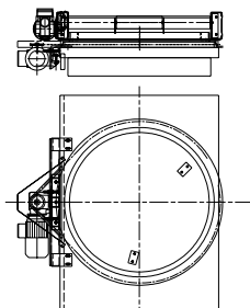
PA1500 – Vridbar rullbana, lågbyggd för montering på lyftbord
