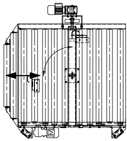
PA1500 – Vridbar rullbana, lågbyggd med hjul, dubbla stödrullar
