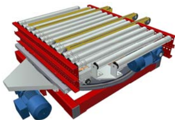
AX100 – Vridmodul med rullbana och vinkelväxel
