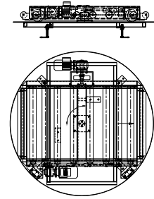
PA1500 – Vridbar rullbana, lågbyggd med hjul rullande på stålskiva
