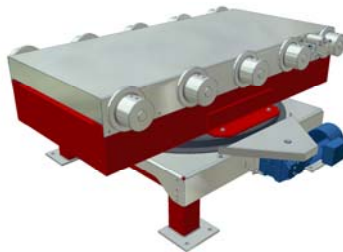
Flänshjulbana – Vridbar flänshjulbana. 3000 kg
