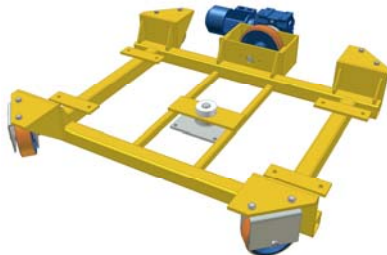
PA1500 – Vridmodul, lågbyggd med hjul
