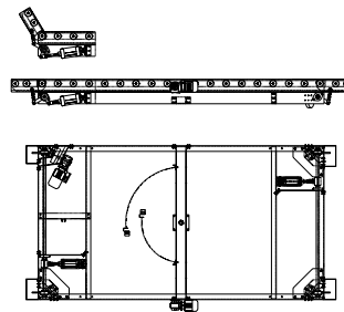
PA1500 – Vridbar rullbana lågbyggd med hjul, uppfällbara ändar. TH 350 mm
