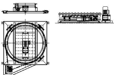
AX100 – Vridbar rullbana, lågbyggd. TH 260 mm
