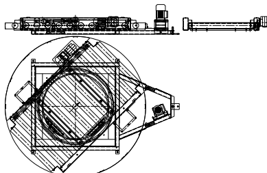
PA1500 – Vridbar rullbana, lågbyggd. TH 160 mm
