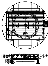
PA1500 – Vridbar rullbana, tre stödrullar per sida
