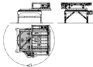
FR100 – Vridbar rullbana med elektrisk rörelse
