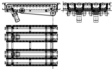
AX100 – Vinkelväxel rem, 6-strängad
