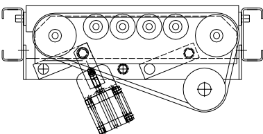
AX100 – Vinkelväxel rem, lågbyggd. TH 260 mm
