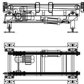
PA1500 – Vinkelväxel, dubbel, 1/2" kedja
