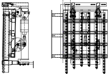
PA1500 – Vinkelväxel, tiltande hjulister, 6-strängad
