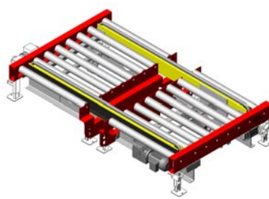
PA1500 – Vinkelväxel, dubbel Typ DV *
