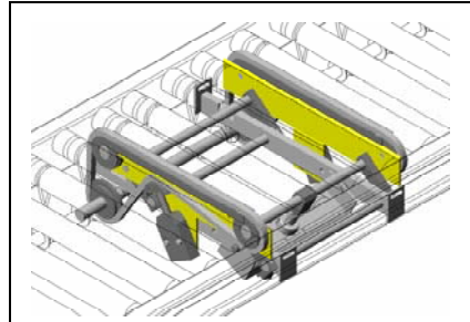
AX100 – Vinkelväxel kedja, enkel Typ VK *
