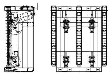
PA1500 – Vinkelväxel, tiltande rullister, 3-strängad
