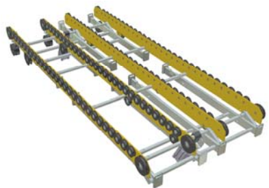
AX100 – Vinkelväxel kedja, dubbel, 4-strängad
