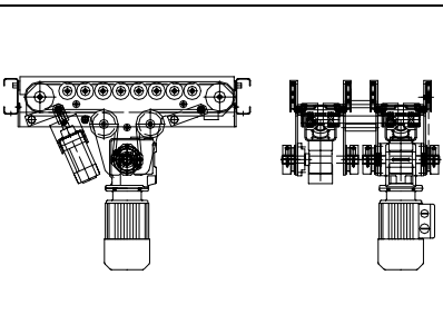
AX100 – Vinkelväxel rem, 4-strängad, separatdriven
