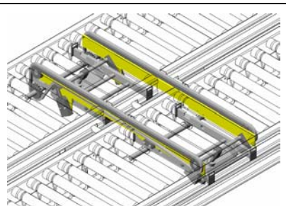
AX100 – Vinkelväxel kedja, dubbel Typ VK *
