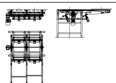
FR100 – Vinkelväxel kuggrem, separatdriven, 3-strängad
