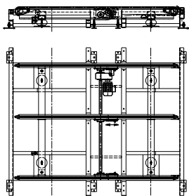
PA1500 – Vinkelväxel, lågbyggd dubbel, 3-strängad med bälgcylindrar
