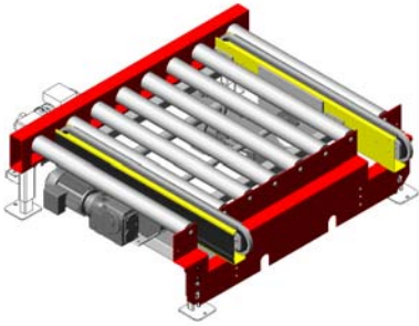
PA1500 – Vinkelväxel, enkel Typ EV *
