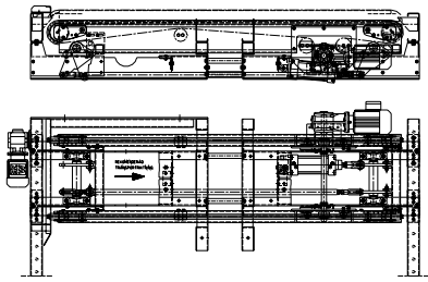
PA1500 – Vinkelväxel, dubbel för 1/2-pall
