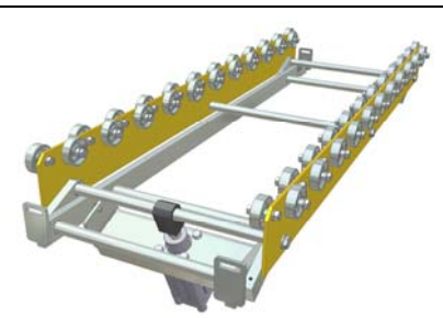
AX100 – Vinkelväxel, hjullist
