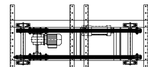
KE500 – Vinkelväxel kedja, dubbel
