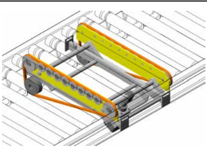
AX100 – Vinkelväxel rem, enkel Typ VR *
