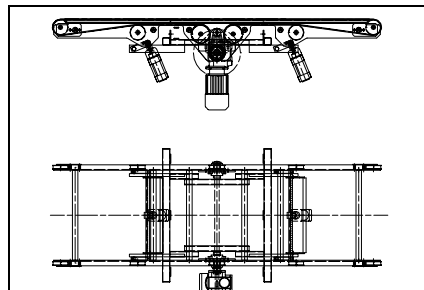
FR100 – Vinkelväxel kuggrem, separatdriven
