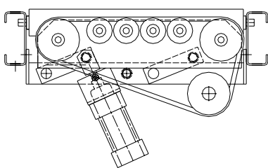
AX100 Rostfritt – Vinkelväxel rem, enkel
