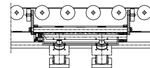
AX100 – Vinkelväxel hjullinjal, enkel, lågbyggd. TH 260 mm
