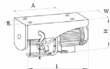
Svängarm/ Rotary hoist frame - SB A
